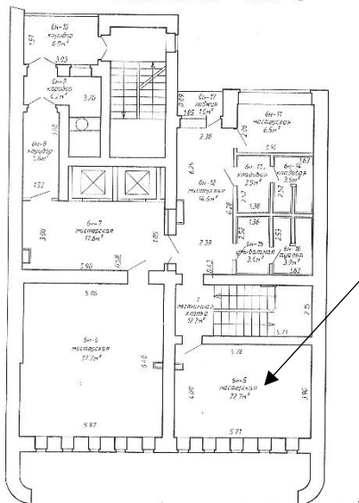
Поздний план (секция/подъезд) - Этаж - 2
